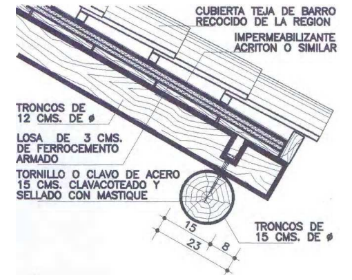
DETALLE CORTE DE LA CUBIERTA
